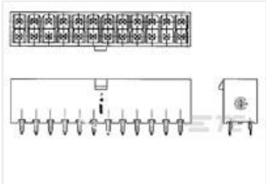
TE 产品编号2-1586037-2 22P VERT HDR VAL-U-LOK V2
