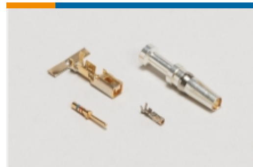
连接器端子(108)
