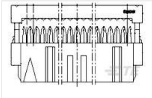
TE 产品编号4-215882-0 40 WAY BLACK MK II RECP
