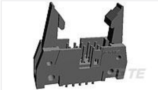
TE 产品编号5499206-6 A/L UNIV HDR 26P VERT LAT
