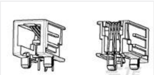
TE 产品编号1-1705949-1 Modular Jack SE, 4/4, Gold flash
