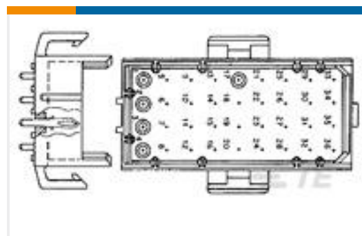
TE 产品编号2-640506-4 36P MR HDR ASSY VO LF
