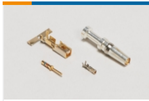
连接器端子(4)
