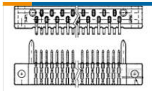
TE 产品编号3-582308-1 47 AMP BLADE HDR ASSY
