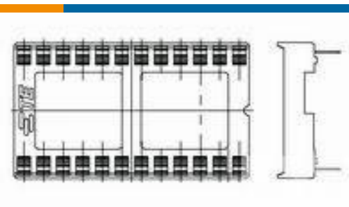
TE 产品编号1-2199299-2 28P,DIP SKT,600 CL,LDR,PB FREE
