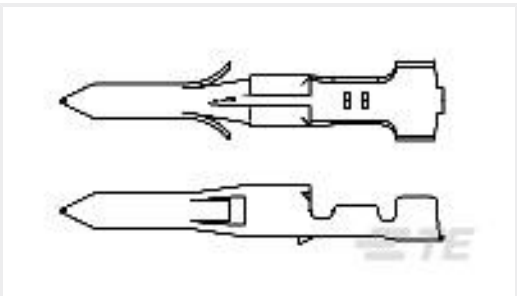
TE 产品编号794018-1 .062 CP&S PIN PTPBR L/P 30-24
