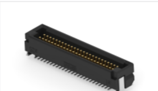
TE 产品编号294139-E DRCQ 0,80 50 M 2 SMD M1 137 E009 176 GU-
