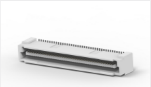
TE 产品编号 CAT-313-PCB80 自由高度插头连接器：板对板, 垂直, 80, 0.8mm
