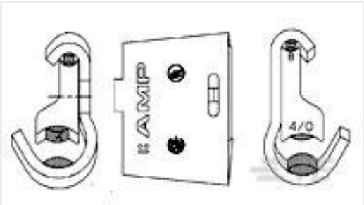
TE 产品编号83623-5 MINIWEDGE,LRG SL,3/0-#10,12,14
