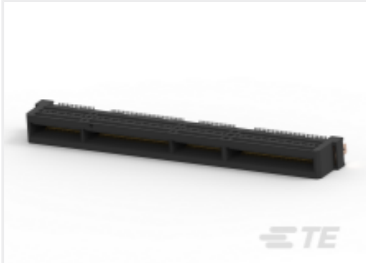
TE 产品编号 2333799-1 RCPT ASSY, VERT, 168 POS, SLIVER 2.0
