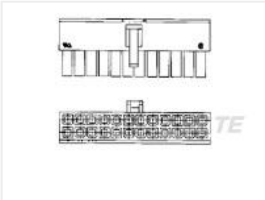
TE 产品编号2-794954-2 22P RCPT VAL-U-LOK V2
