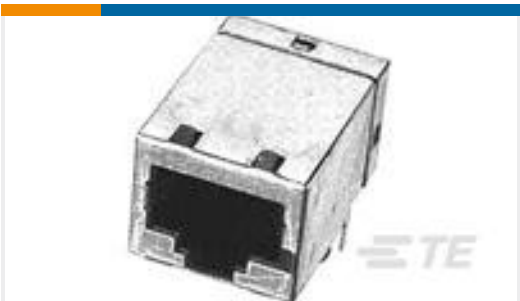
TE 产品编号1-1734580-3 MOD-Jack,RJ45, 10P10C, SHD LP, 30u" Au
