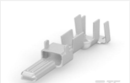
TE 产品编号4-1971784-2 PTL TAB CONTACT LP, 16-19 AWG, 2X22
