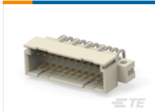
TE 产品编号384226-E STVC/3 20 M AC WV 4-00 0606 * * 247 E007
