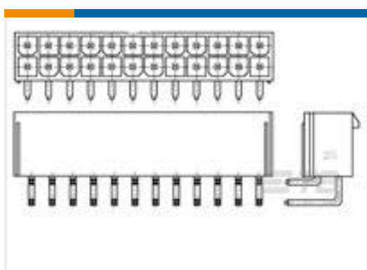
TE 产品编号1-1586041-4 14P VAL-U-LOK R/A HDR V2
