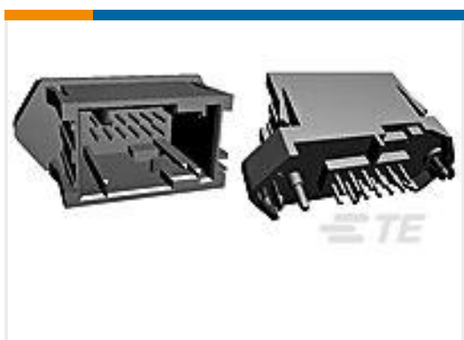
TE 产品编号1379114-3 12pos MQS .63 header 180deg
