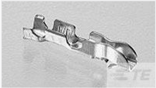
TE 产品编号 170263-1 EIS CONTACT
