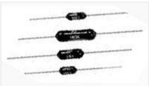
TE 产品编号1879663-1 H8 107R 0.1% 15PPM
