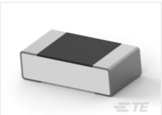
TE 产品编号3-2176372-4 RQ 0603 110K 0.1% 10PPM 5K RL
