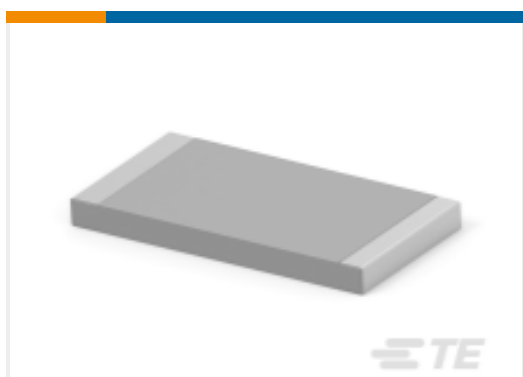
TE 产品编号2-2176331-1 CRGP 2512 470R 1%
