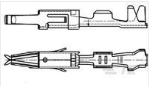
TE 产品编号 963711-2 MICRO TIM RECEPTACLE CONTACT
