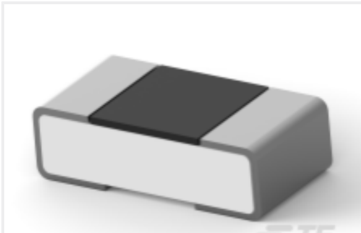
TE 产品编号8-2176363-3 RQ 0402 3K09 0.1% 10PPM 5K RL
