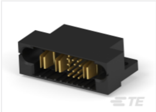
TE 产品编号1-6600132-5 MBXL R/A HDR DB 2ACP + 12S + 1P
