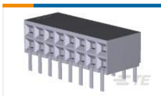
TE 产品编号 1-5535512-8 16 MODII HORZ DR CE EESS .100
