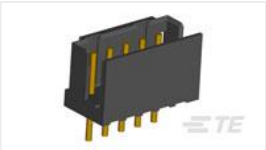
TE 产品编号820671-000 222K132-3/42-0
