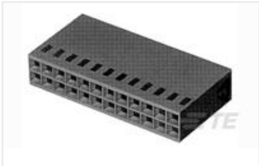
TE 产品编号1-87456-1 16 MODIV HSG COMP DR .100CL
