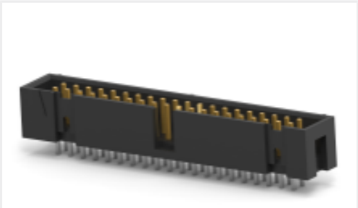
TE 产品编号 1-1761681-3 IDC LOW PRO HDR 40P VERT HT BLACK
