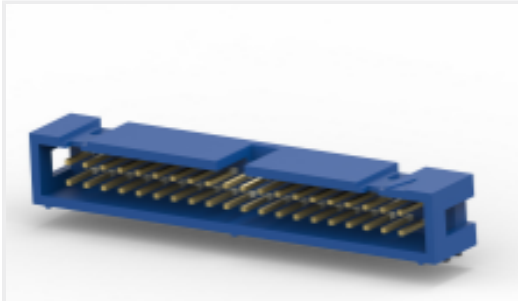
TE 产品编号 3-1761605-3 IDC LOW PRO HDR 40P RA BLUE
