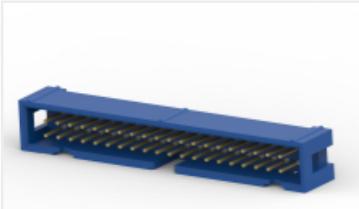
TE 产品编号 3-1761603-3 IDC LOW PRO HDR 40P VERT BLUE
