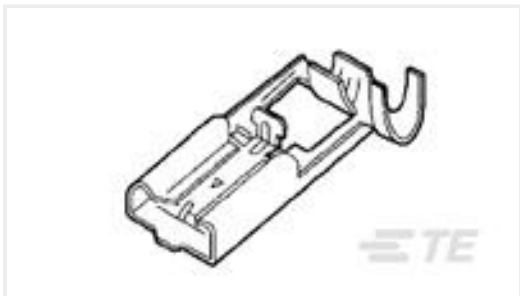
TE 产品编号172795-1 PL 312 FLAG REC 20-14 0.32 X 24.9 PTPBR
