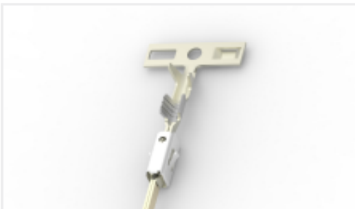
TE 产品编号2141882-3 TAB A 1.6x0.6 CONTACT CS SRC Au
