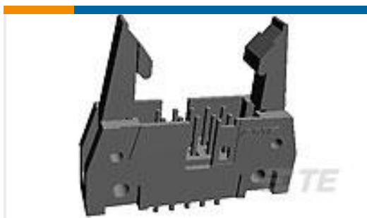
TE 产品编号2-5499206-4 A/L UNIV HDR 20P VERT LG LAT B
