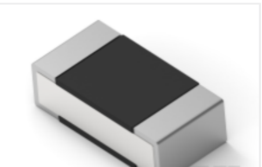
TE 产品编号2176313-9 RP 1E 0.1W 162K 0.1% 25PPM 1K RL
