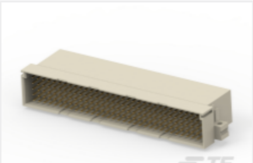
TE 产品编号384299-E STVE 160 M ABCDE VVVV 4-00 0606 ** 247
