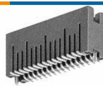
TE 产品编号 5-104693-8 80 50/50 HDR DRST SFMNT.390 SN
