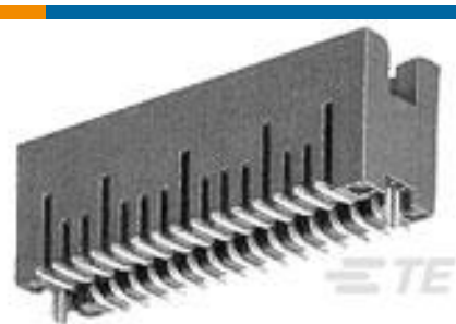
TE 产品编号 5-104656-8 80 50/50 HDR DRST SFMNT.320 SN
