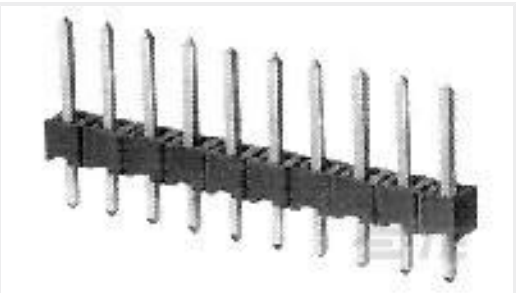
TE 产品编号826926-4 4P AMPMODU II STIFT LEI
