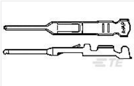
TE 产品编号170430-1 EI PIN LP 170377-1 LP
