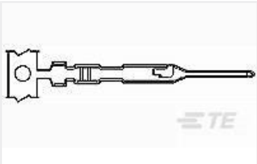
TE 产品编号5-104505-4 MTE PIN 22-26 AWG PLTD
