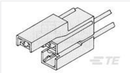
TE 产品编号360010-1 187 FASTON HSG.,REC.,3 POS, NATRUAL
