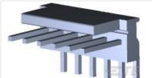
TE 产品编号 640455-6 06P MTA100 HDR ASSY SQ R/A POL
