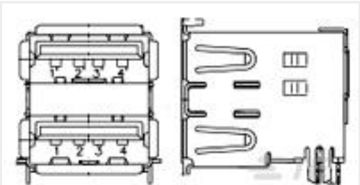
TE 产品编号 1734510-2 MINI USB, TYPE B, R/A, T/H
