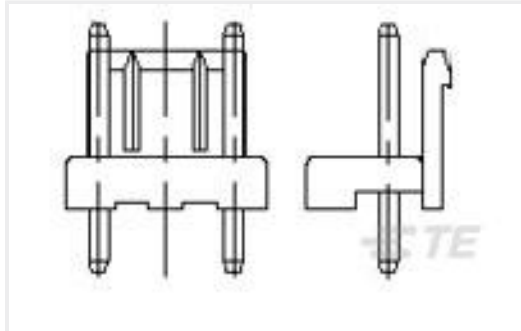
TE 产品编号1744103-1 3.96 EPHDR ASSY 3P OMIT #2 PIN
