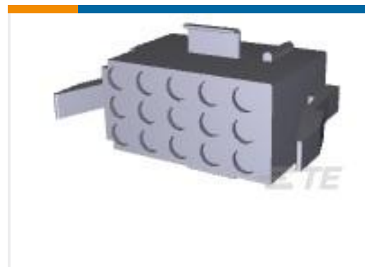
TE 产品编号1-480323-0 15P CMNL PLUG HSG P/M NATL
