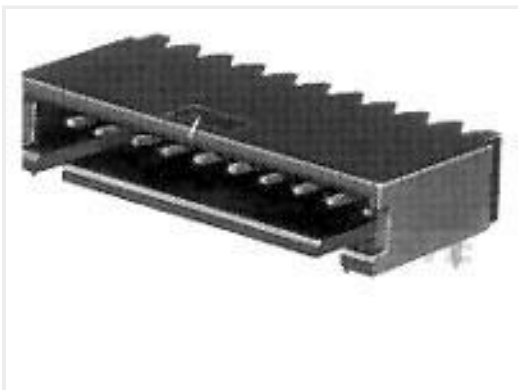
TE 产品编号 5-102523-1 04 MODII HDR SRRA SHRD .100CL
