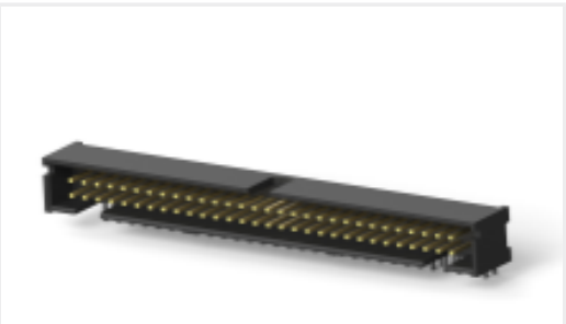
TE 产品编号 1-5103311-2 A/L LOW PRO HDR 60P RA BLACK
