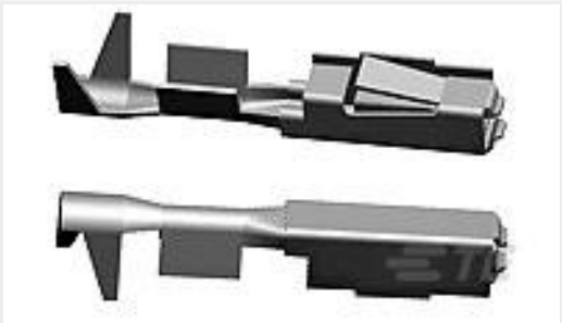
TE 产品编号5-965906-5 MQS0,63 Au rec LL EDS 0,5-0,75
