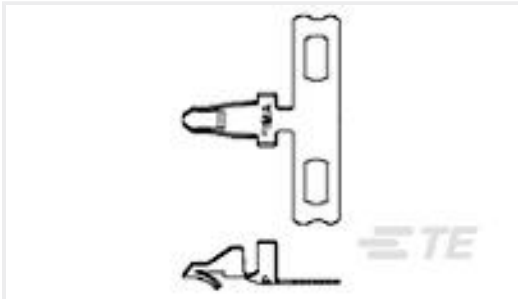
TE 产品编号350566-3 MINI AMP-IN 22-18 PTPBR
