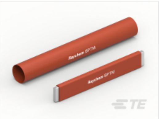
TE 产品编号040337-000 BPTM-50/20-A/U(B50)
