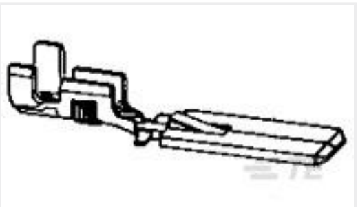
TE 产品编号280074-2 FF 375 TAB 6-10MM2 PTBR
