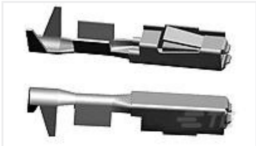
TE 产品编号5-962885-5 MQS0,63 Au rec LL EDS 0,2-0,35
