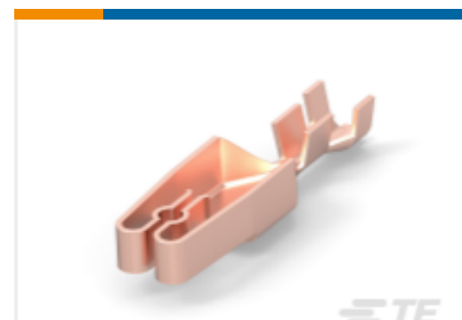
TE 产品编号 530517-1 CONT.HIGH CURRENT STRIP
